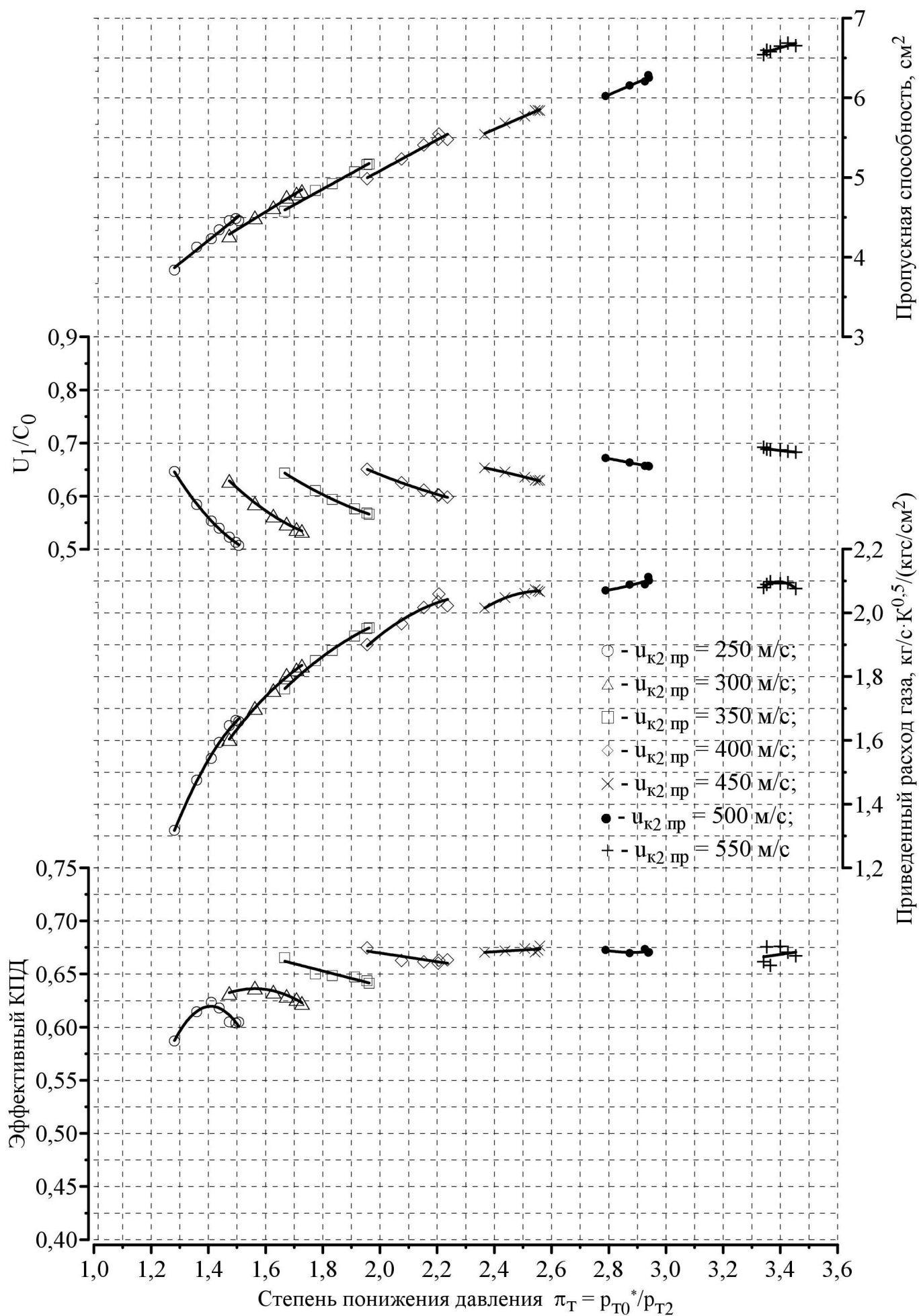
Рисунок - Характеристики турбины ТКР 60-14 d_{T1} = 60 мм, d_{T2} = 50 мм, z = 11 , d_B = 8,5 мм, F_T = 10 см 2 , корпус однозаходный с перепуском, t_{T0} = 650 °С
