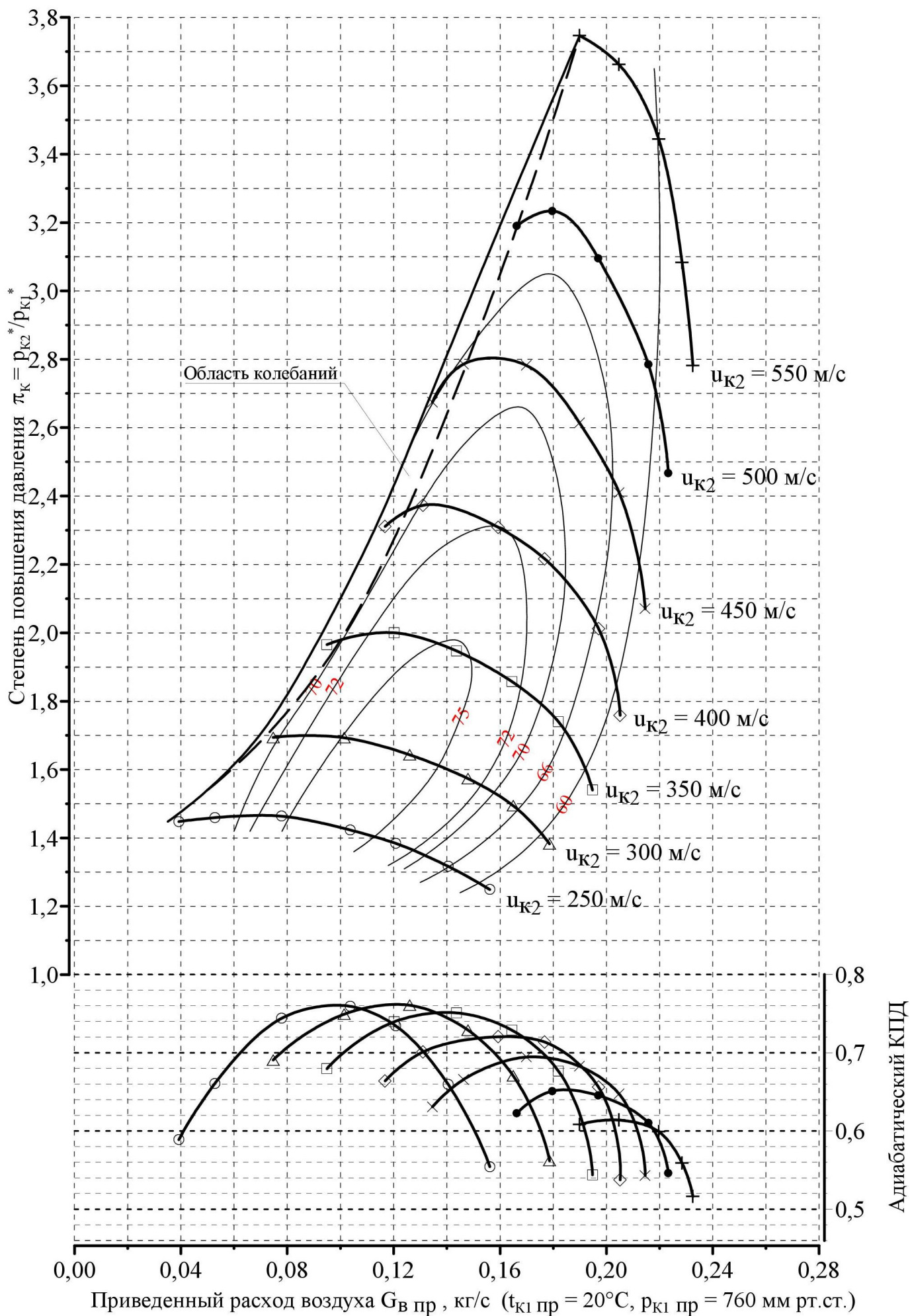
Рисунок - Характеристики компрессора ТКР 60-14 d_2 = 65 \text{ мм} , d_1 = 43,5 \text{ мм} , d_0 = 14,7 \text{ мм} , z = 12(6) , b_2 = 4,5 \text{ мм} , b_4 = 4,0 \text{ мм} , d_4 = 95 \text{ мм}
